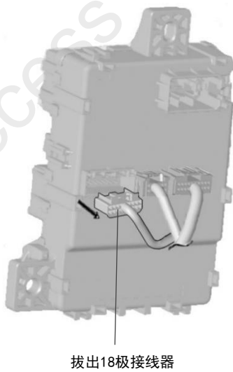
【保险丝盒背视图】
