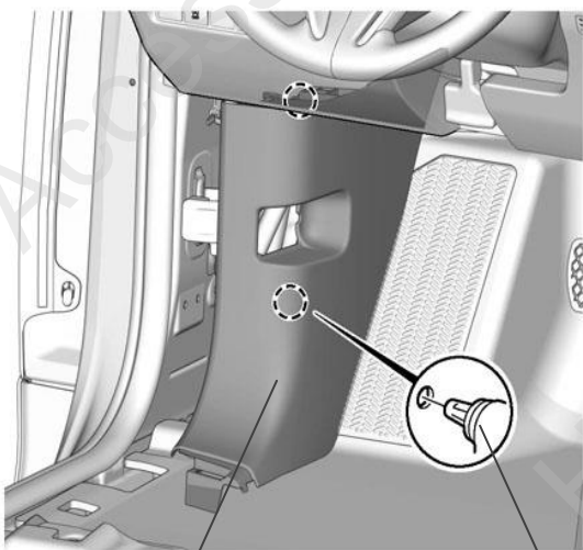
左前侧饰板 夹扣 (2)
