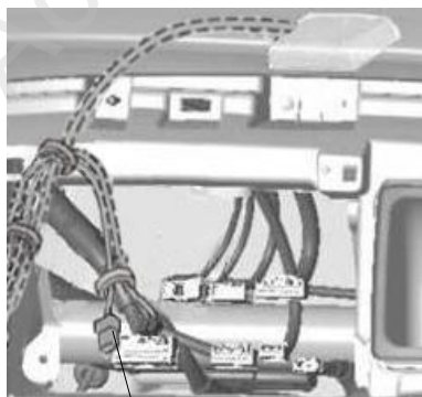
USB连接器
