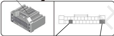
车辆：紫色导线 用品：白色导线
