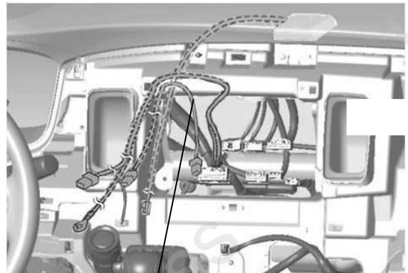
绿色端：连接控制单元 灰色端：连接 DA
