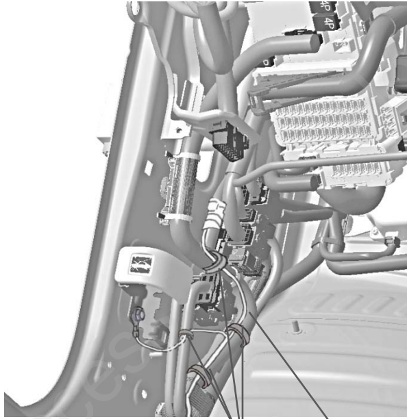
车辆线束 线束胶带 (4)
