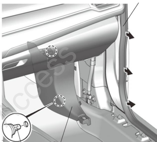
夹扣 (2) 右前侧饰板
