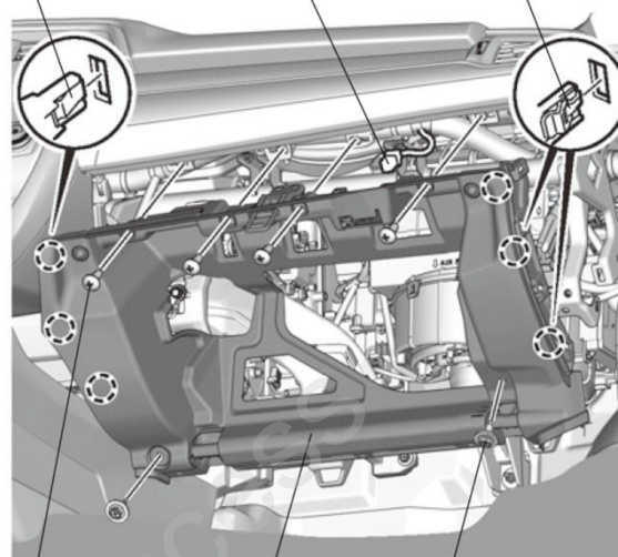
自攻螺丝 (4) 手套箱护板 螺栓 (2)
