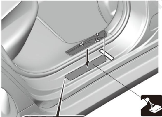
右后门边踏板饰条 车辆面板 R角 〈截面图〉
