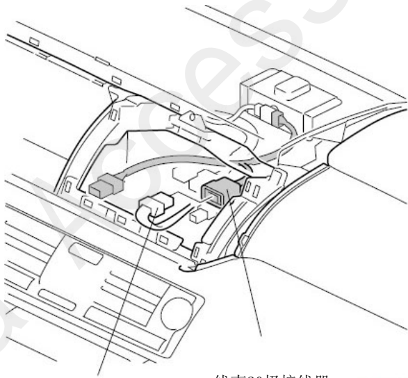
线束20极接线器 QAN2206AE
