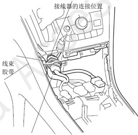
车辆线束
