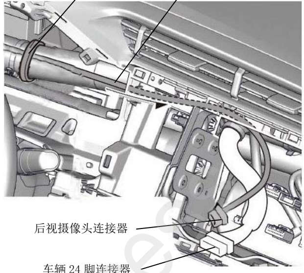
车辆 24 脚连接器
