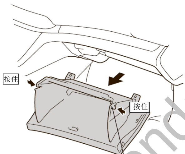
限位器 (2)
